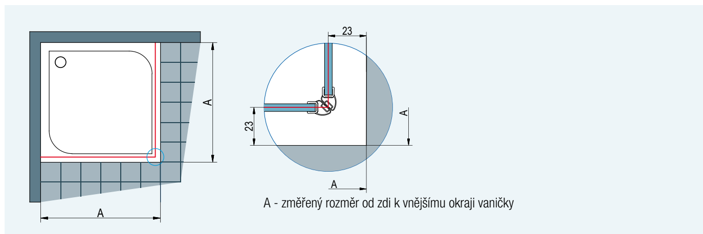
Obr. 1: Při montáži na vaničku je odsazení 23 mm stejné pro všechny typy řady ANNEA.
